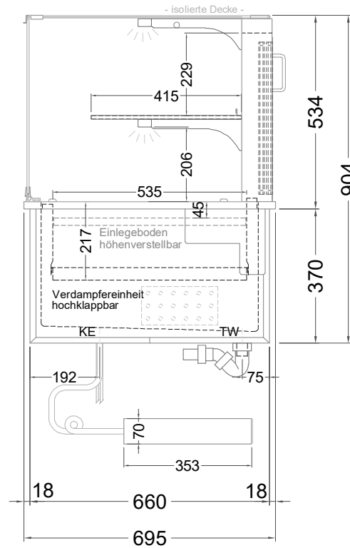
(Seitenansicht)
