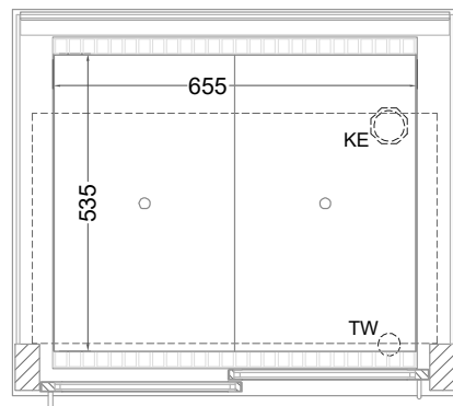
(Grundriss)
