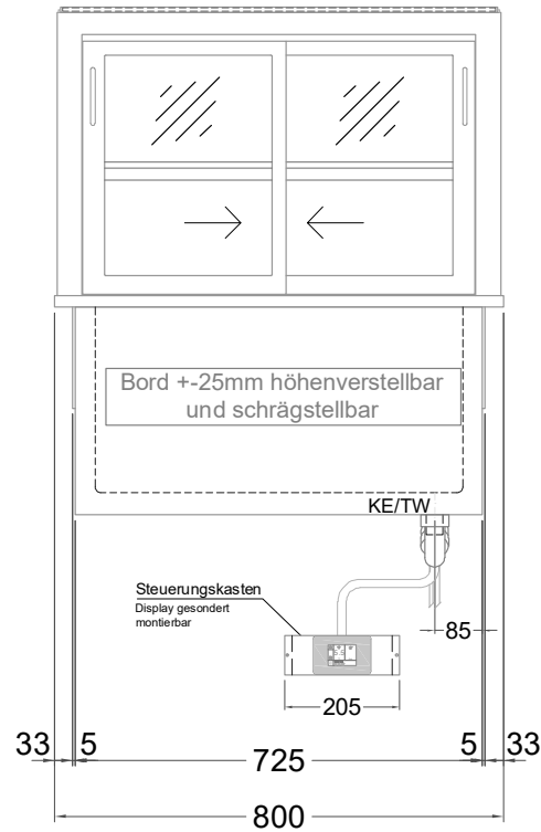
(Bedienseite)
