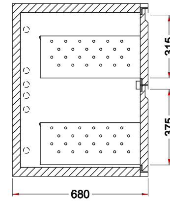
Schnitt L1
