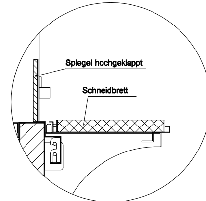
(Detail Spiegelsystem)
