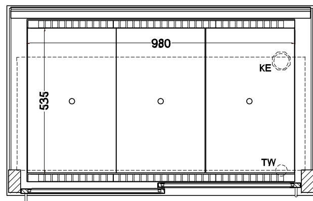
(Grundriss)
