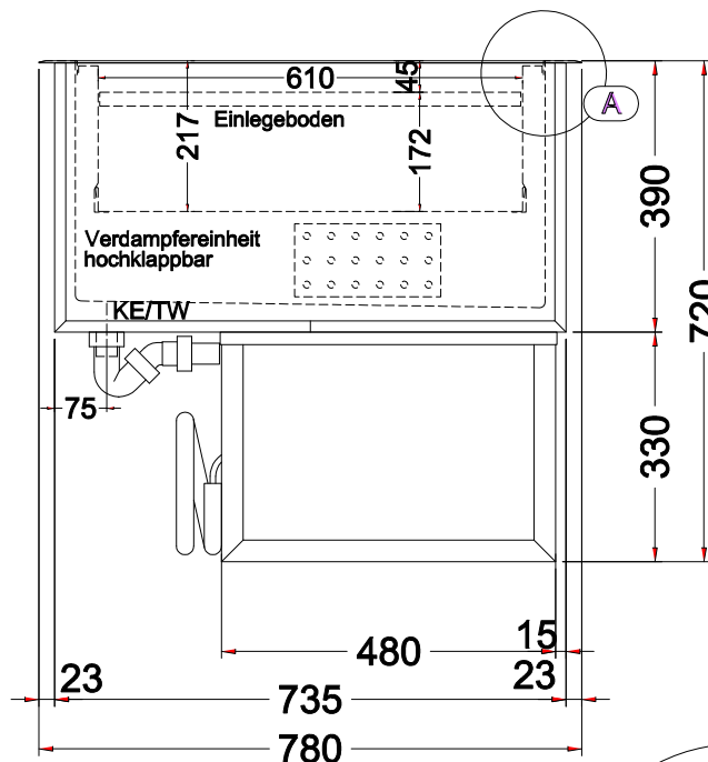
(Seitenansicht)
