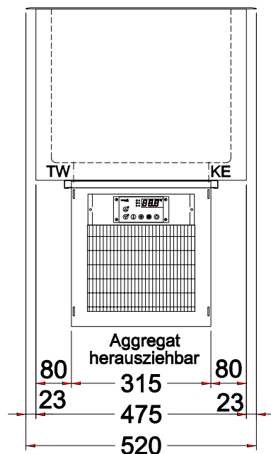
(Bedienseite)
