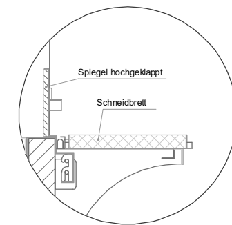
(Detail Spiegelsystem)
