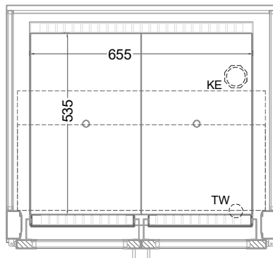
(Grundriss)
