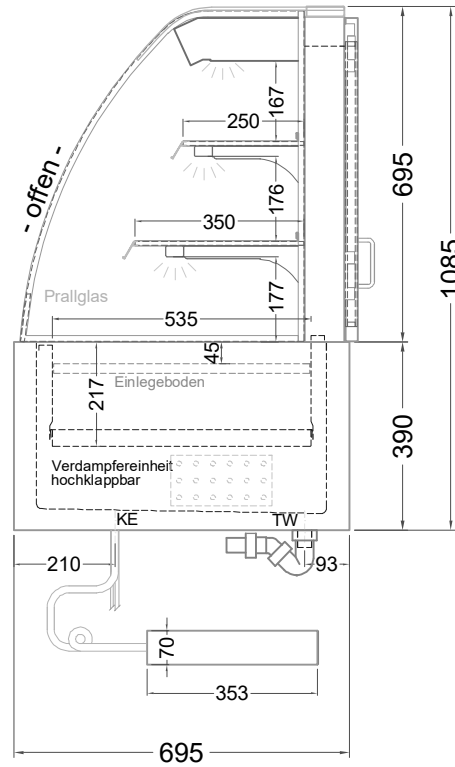
(Seitenansicht)
