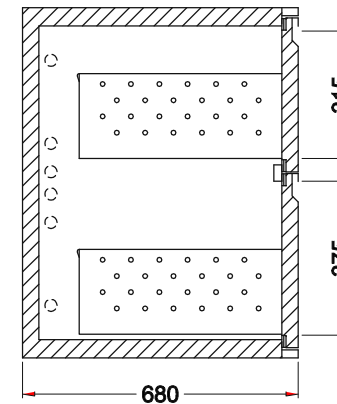
Schnitt L1
