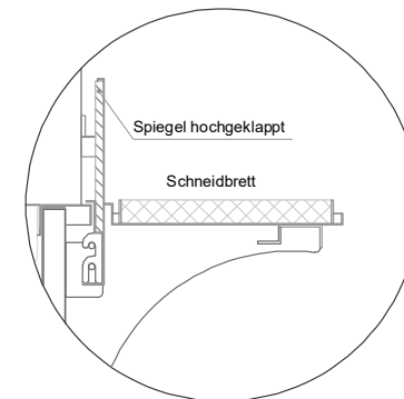
(Detail Spiegelsystem)
