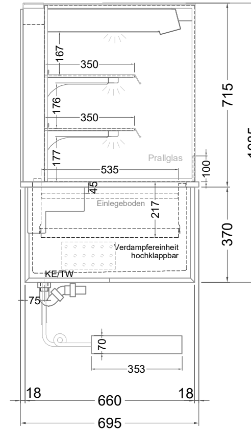
(Seitenansicht)
