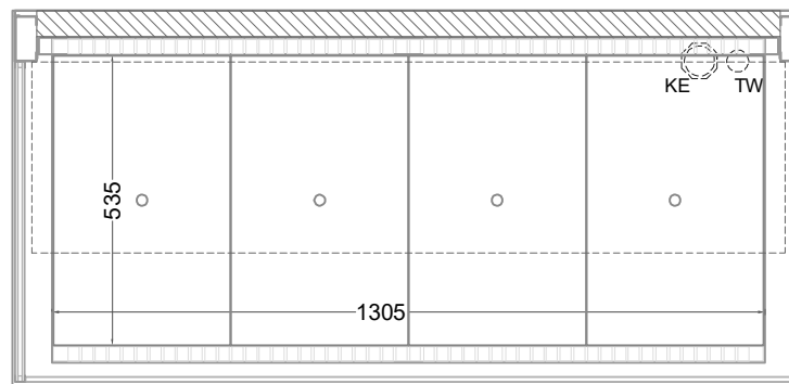
(Grundriss)
