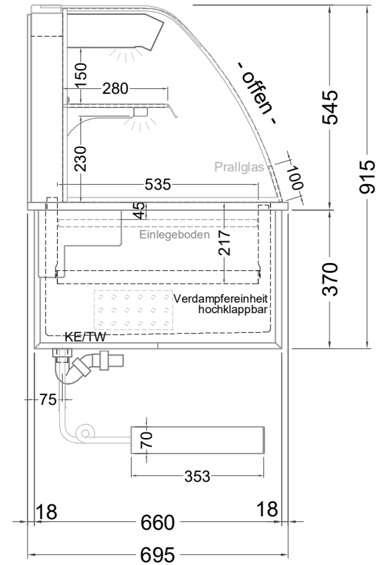
(Seitenansicht)
