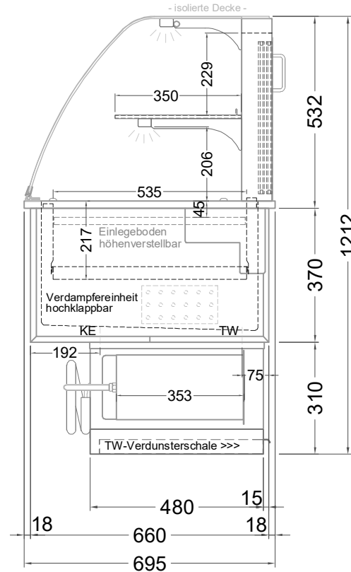
(Seitenansicht)
