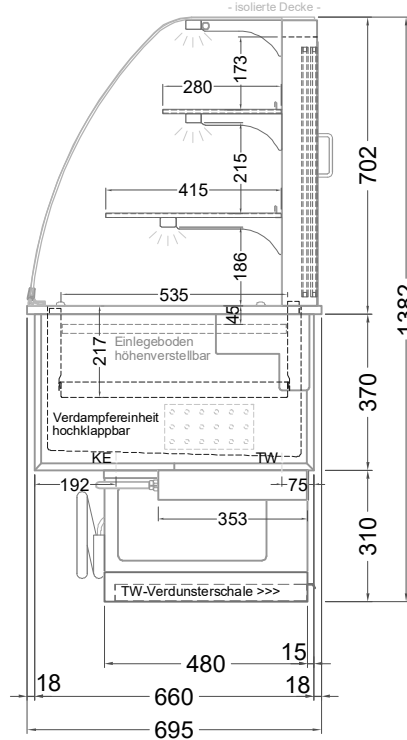
(Seitenansicht)
