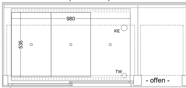
(Grundriss)
