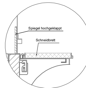
(Detail Spiegelsystem)
