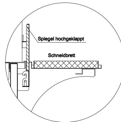
(Detail Spiegelsystem)
