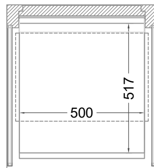
(Grundriss)
