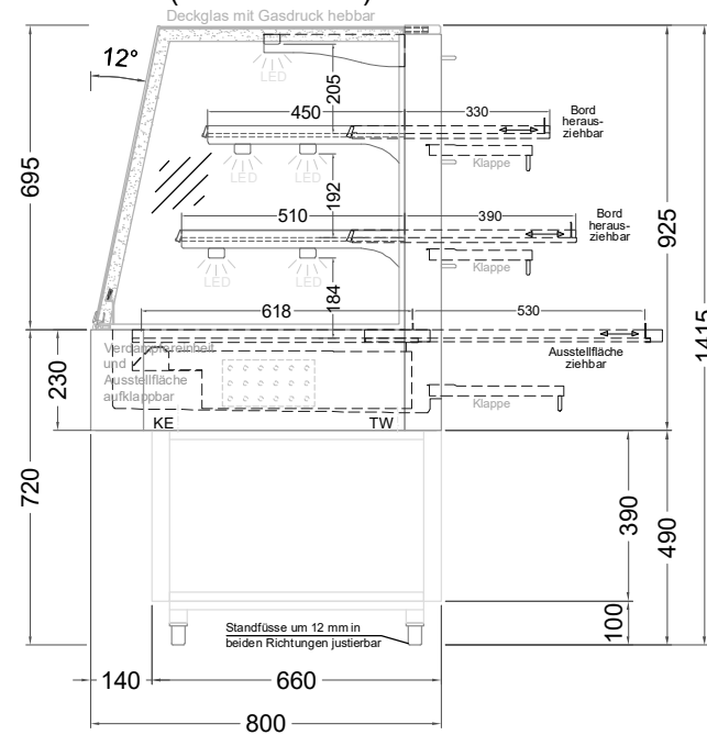
(Seitenansicht)
