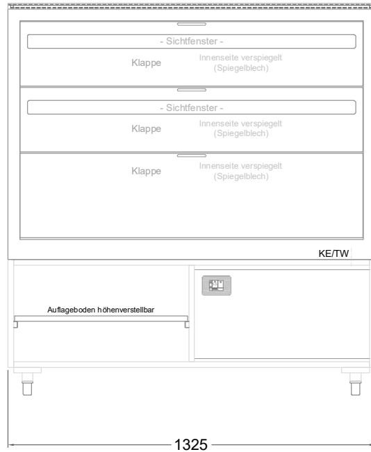
(Bedienseite)
