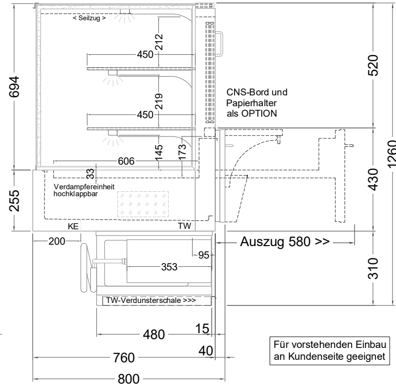
(Seitenansicht)
