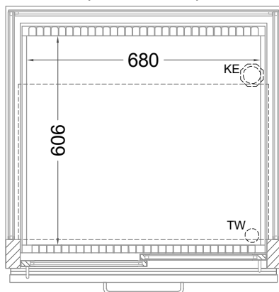
(Grundriss)
