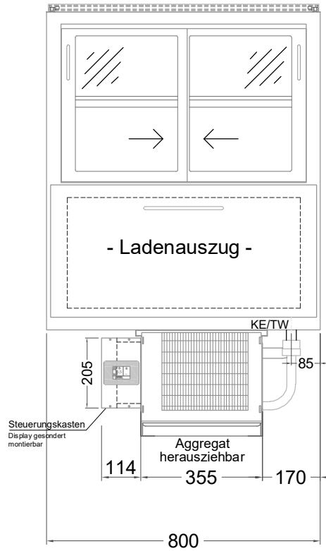
(Grundriss)
