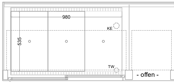
(Grundriss)
