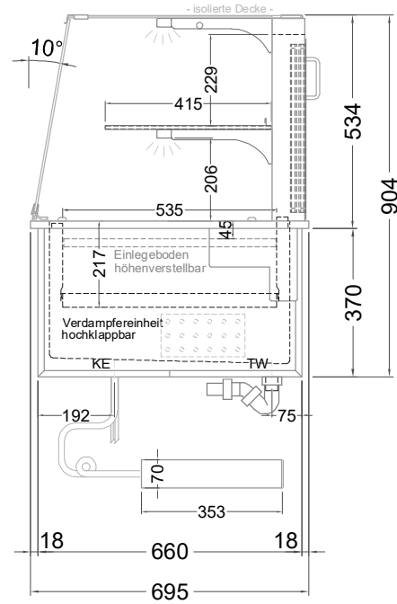
(Seitenansicht)
