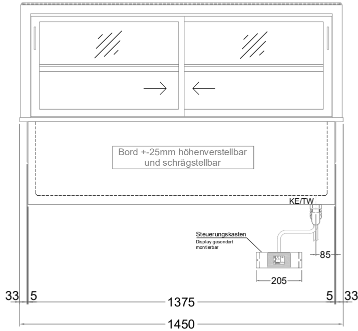
(Bedienseite)
