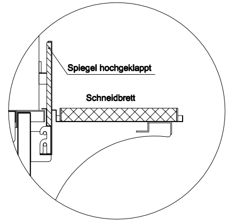
(Detail Spiegelsystem)
