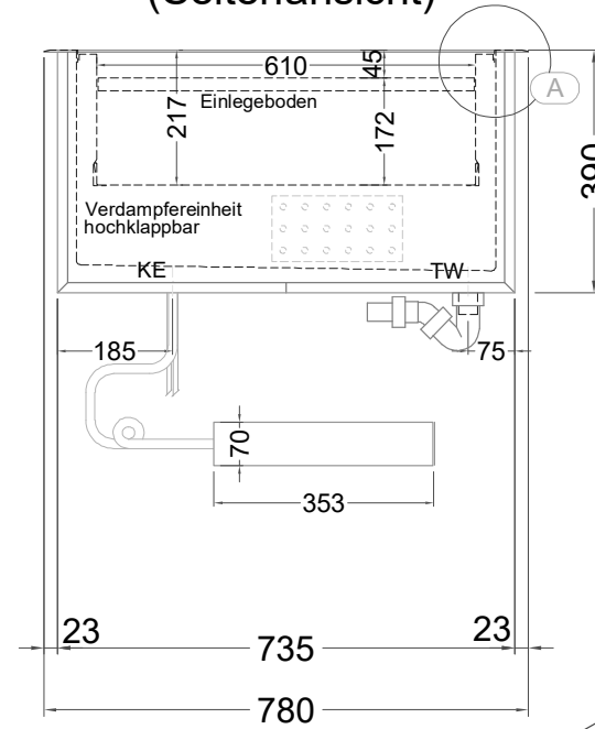
(Seitenansicht)
