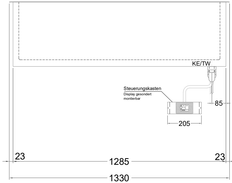
(Bedienseite)
