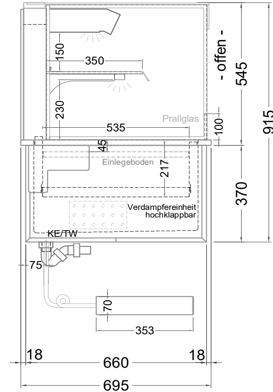
(Seitenansicht)
