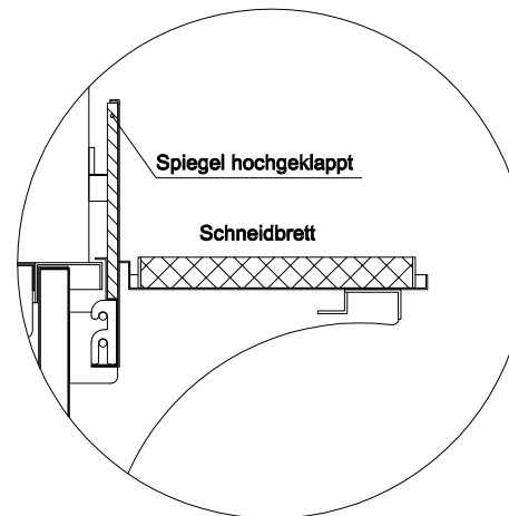
(Detail Spiegelsystem)
