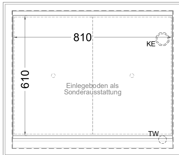
(Grundriss)
