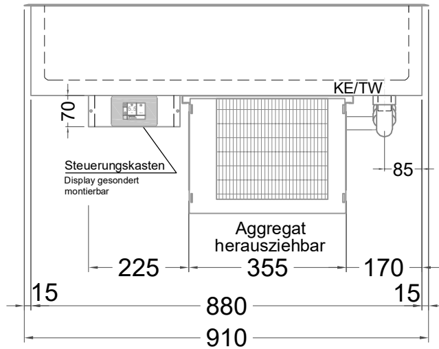
(Bedienseite)
