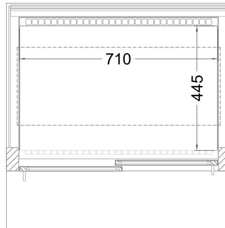
(Grundriss)
