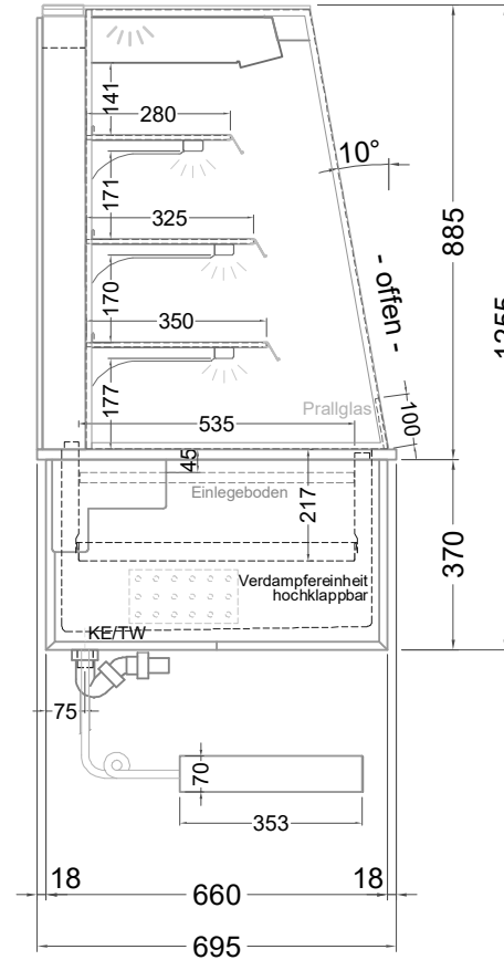
(Seitenansicht)
