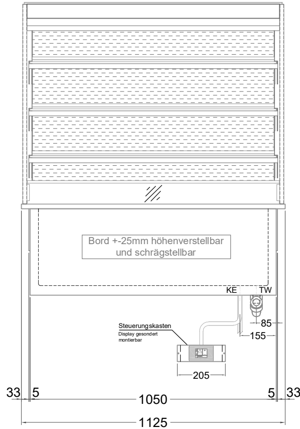
(Vorderseite)
