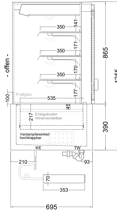
(Seitenansicht)
