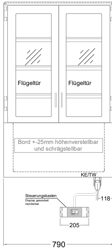
(Bedienseite)
