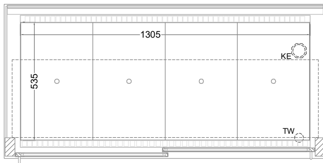
(Grundriss)
