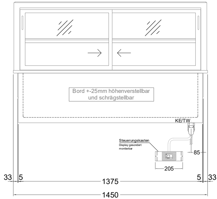
(Bedienseite)
