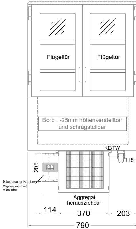
(Bedienseite)
