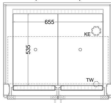
(Grundriss)
