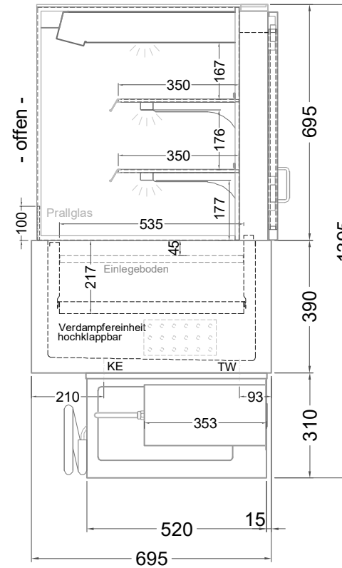
(Seitenansicht)
